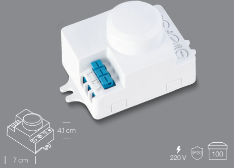
ZMR-536 360° SLIM SIVA ÜSTÜ SENSÖR
