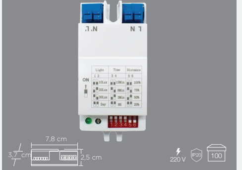
ZMR-535 180° HAREKET SENSÖRÜ
