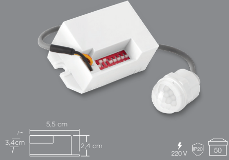
ZMR-532 10A 360° SIVA ALTI SENSÖR
